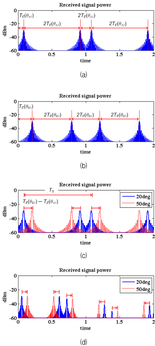
그림 11. 양방향 섹터 및 6단 라스터 스캔 레이더 수신 신호 (a) \theta=20^\circ 일 때의 양방향 섹터 스캔 레이더 수신 신호, (b) \theta=50^\circ 일 때의 양방향 섹터 스캔 레이더 수신 신호, (c) ES 시스템의 위치에 따른 양방향 섹터 스캔 레이더 수신 신호 비교, (d) ES 시스템의 위치에 따른 6단 라스터 스캔 레이더 수신 신호
