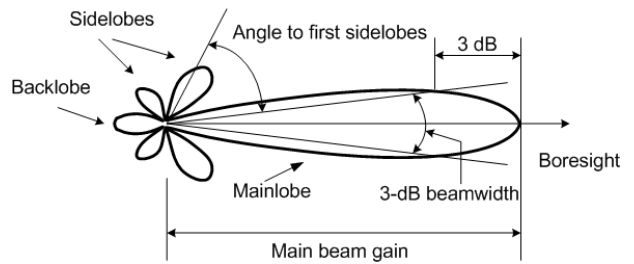
그림 4. 지향성 안테나의 일반적인 방사패턴 Fig. 4. General radiation pattern of a directional antenna.
