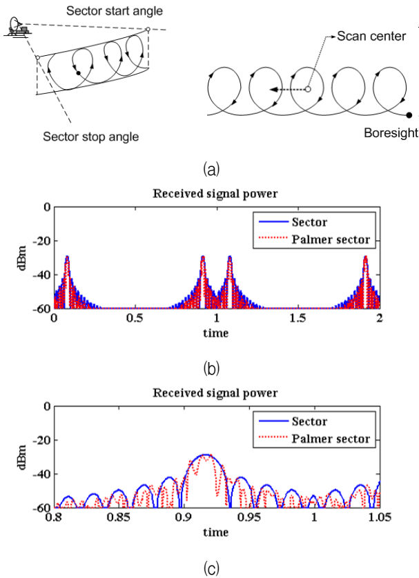
그림 13. 팔머 양방향 섹터 스캔 레이더 수신신호 (a) 조준선의 움직임 (b) 양방향 섹터 스캔 레이더 수신신호와 포락선 비교 (c) 양방향 섹터 스캔 레이더 수신신호와 포락선 확대 비교
