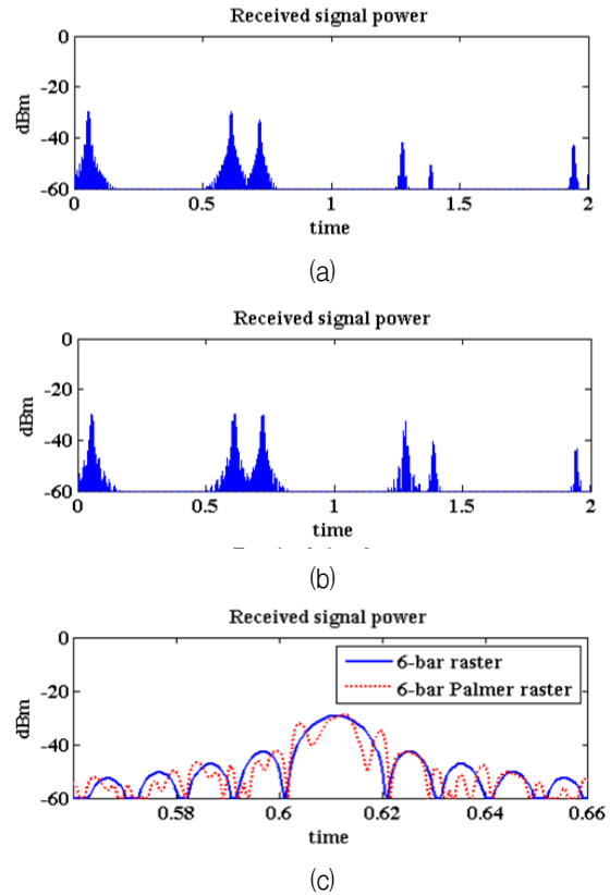
그림 14. 6단 팔머 라스터 스캔 레이더 수신신호 (a) 6단 라스터 스캔 레이더 수신신호, (b) 6단 팔머 라스터 스캔 레이더 수신신호, (c)라스터 및 팔머 라스터 스캔 레이더 수신신호의 세부 형태 비교
