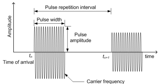
그림 1. ES 시스템에 수신된 레이더 신호 Fig. 1. The received radar signals in an ES system.
