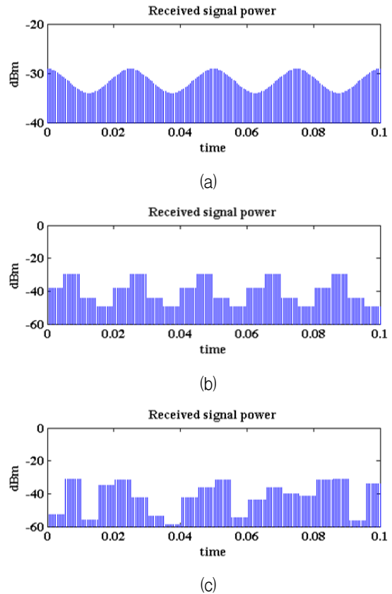
그림 15. 추적 스캔 레이더 수신신호 (a) 원추 스캔 레이더 수신신호 (b)로브스위칭 스캔 레이더 수신신호 (c) 전자로브스위칭 스캔 레이더 수신신호 Fig. 15. Tracking scan radar signals (a) Received conical scan radar signal, (b) Received lobe switching scan radar signal, (c) Received electronic lobe switching scan radar signal.
