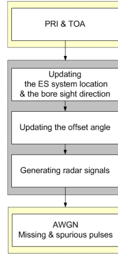
그림 7. 제안된 레이더 수신신호 생성 기법의 블록도 Fig. 7. The block diagram of the proposed radar signal generation method.
