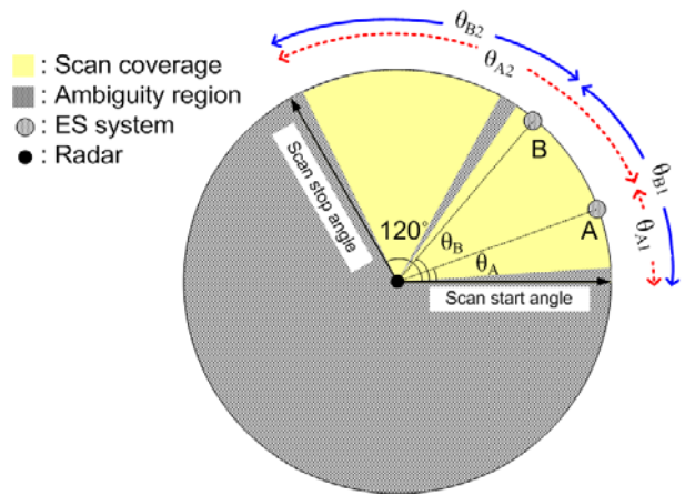
그림 10. 양방향 섹터 및 라스터 스캔 레이더의 조준선 이동
