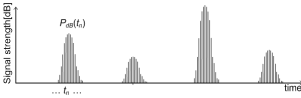
그림 5. 스캔패턴 분석을 위한 레이더 수신신호의 예 Fig. 5. An example of the received radar signal for scan pattern analysis.
