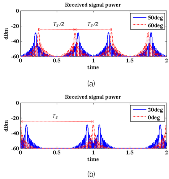
그림 12. 식별모호 영역에서의 레이더 수신신호 특성 (a) 스캔영역의 중앙에서의 레이더 수신신호, (b) 스캔영역 경계에서의 레이더 수신신호
